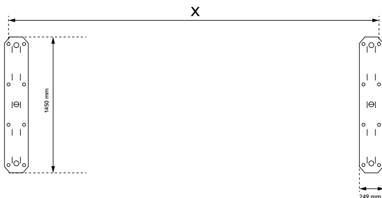
Rys. 4. Rozmieszczenie marek stalowych do montażu carportu Avrii SOL Integra X- odległość zależna od zastosowanych modułów fotowoltaicznych
