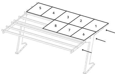
Rys. 21. Poprawna kolejność montażu modułów na konstrukcji
