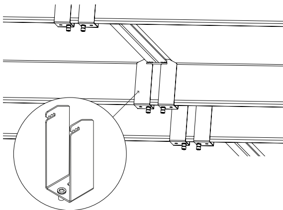
Rys. 24. Mocowanie modułów do konstrukcji carportu
